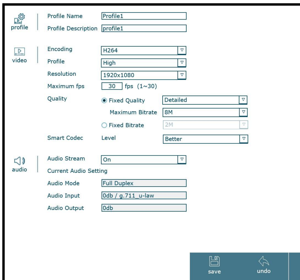
圖 9. 新增/編輯碼流設定檔頁面
